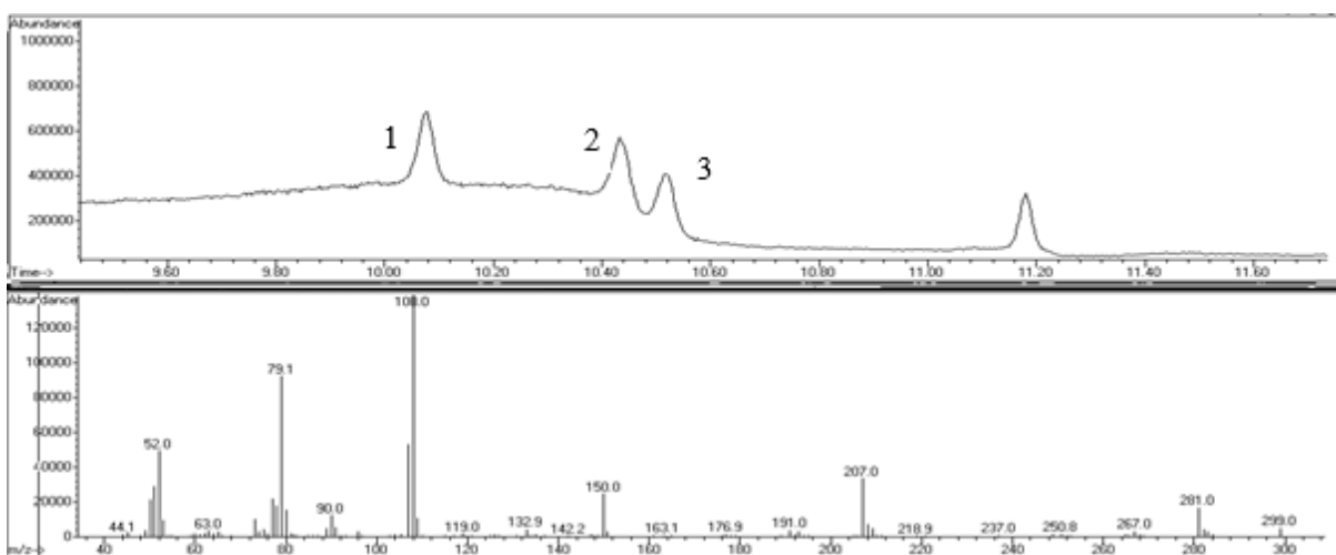
Figura 1: Espectômetro de massas- Modo Scan- orto- cresol
