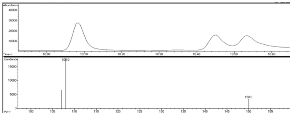
Figura 3: Cromatograma e comportamento dos íons da solução padrão em solvente
