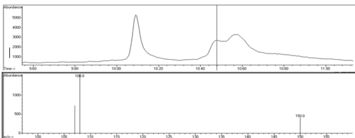
Figura 2: Cromatograma de recuperação de cresóis na matriz solo
